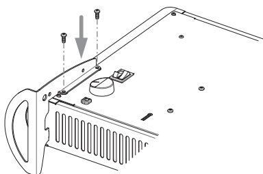
Рисунок 4. Установка опор
