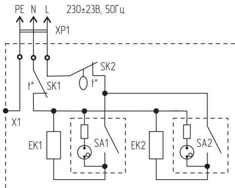
Рисунок 3. Электрическая схема конвектора
